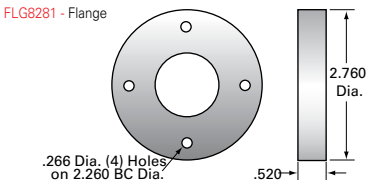
FLG8281 - Flange
