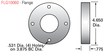
FLG10060 - Flange
