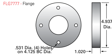
FLG7777 - Flange
