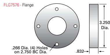
FLG7576 - Flange
