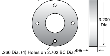
FLG8283 - Flange
