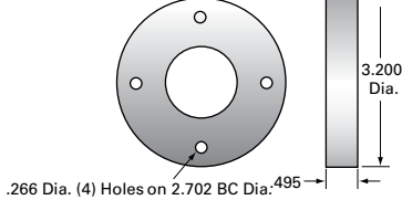
FLG8283 - Flange
