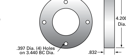
FLG7572 - Flange
