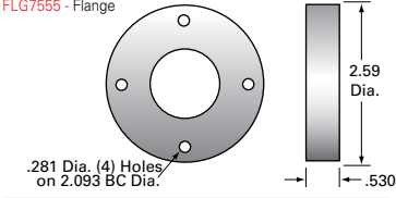
FLG7555 - Flange
