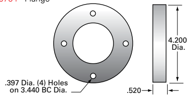
FLG6754 - Flange
